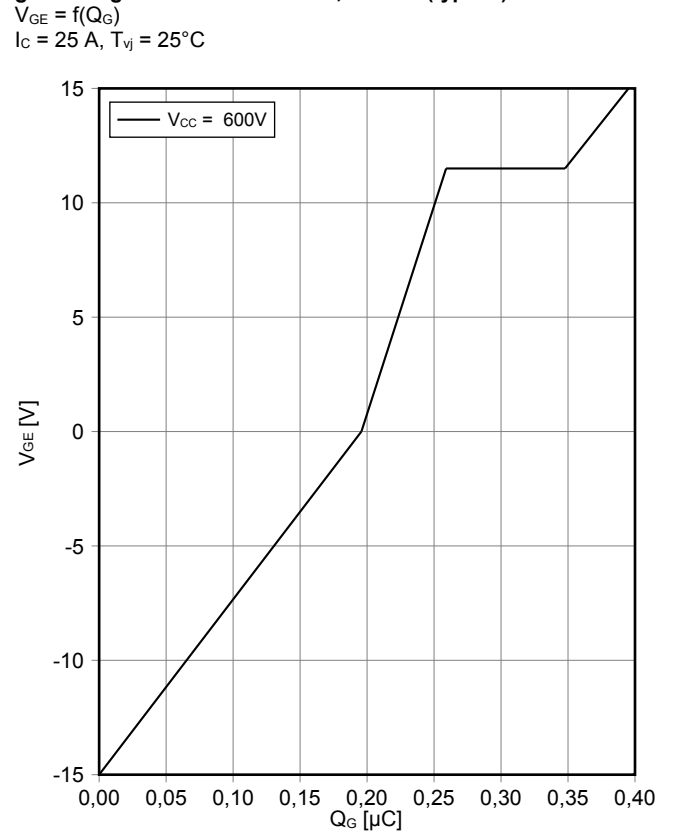
Gateladungs Charakteristik IGBT, Wechselrichter (typisch) gate charge characteristic IGBT, Inverter (typical) V_{GE} = f(Q_G) I_C = 25\text{ A} , T_{vj} = 25^\circ\text{C}
