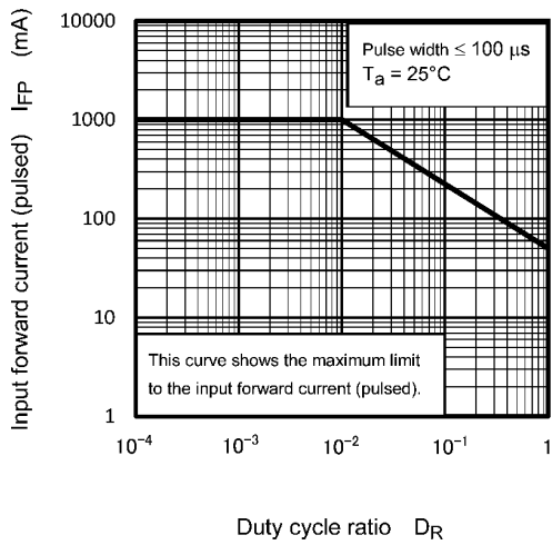
Fig. 11.3 I_{FP} - D_R
