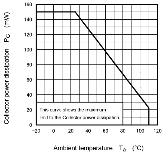
Fig. 11.2 P_C - T_a
