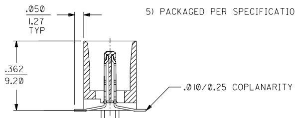
SECTION A-A SCALE 4:1
