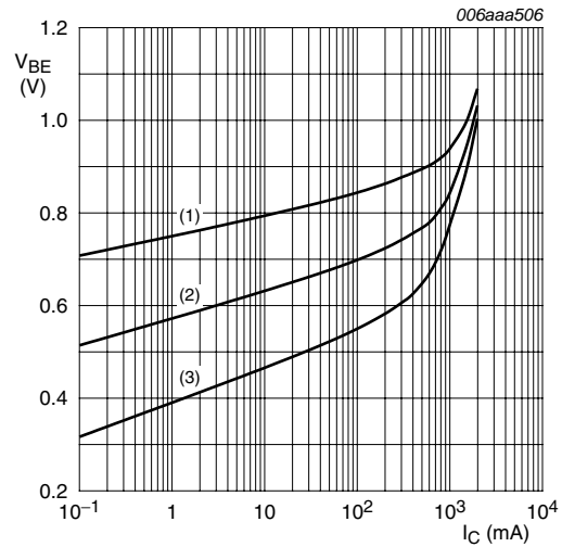
V_{CE} = 5\text{ V} (1) T_{amb} = -55^\circ C (2) T_{amb} = 25^\circ C (3) T_{amb} = 100^\circ C
