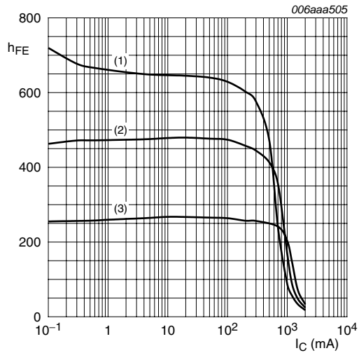
V_{CE} = 5\text{ V} (1) T_{amb} = 100^\circ C (2) T_{amb} = 25^\circ C (3) T_{amb} = -55^\circ C
