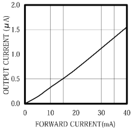
IF VS I o @VR=10V
