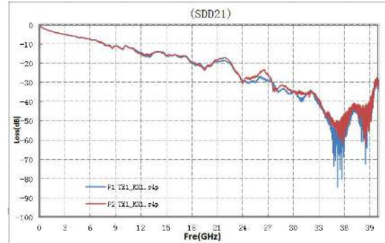
SFP28 30AWG 2M
