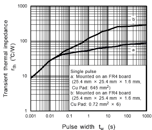
Fig. 7.3.1 r_{th} - t_w
