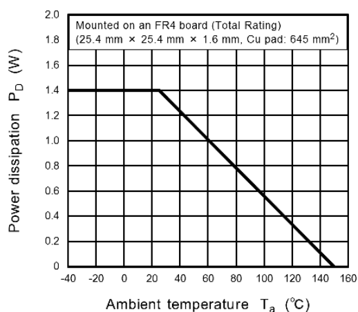
Fig. 7.3.2 P_D - T_a
