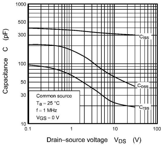
Fig. 7.1.9 C - V_{DS}
