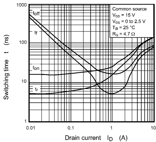
Fig. 7.1.10 t - I_D
