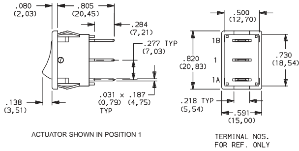
D102J12S215QA SPDT
