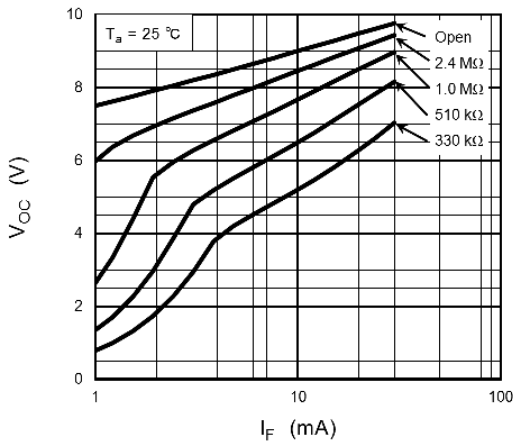
Fig. 12.3 V_{OC} - I_F
