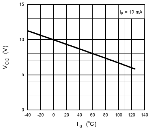
Fig. 12.5 V_{OC} - T_a
