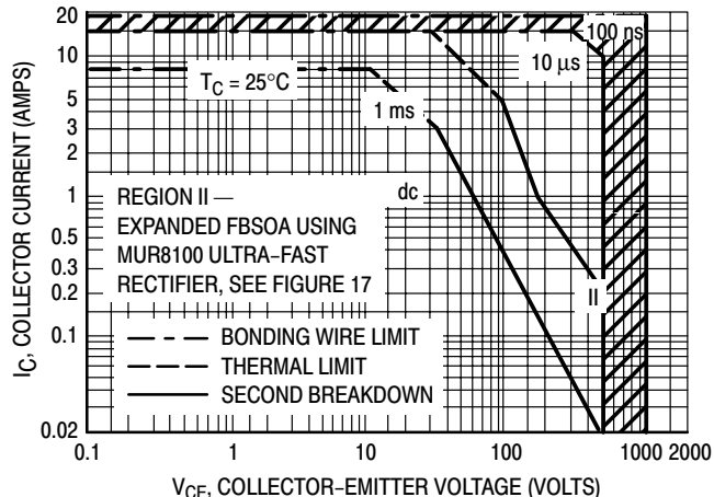
a. MJH16006A
