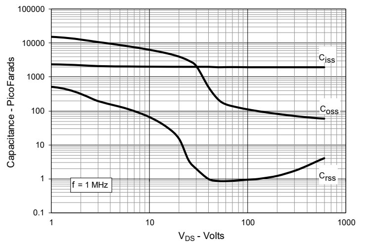
Fig. 12. Capacitance
