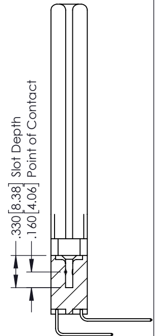
SECTION A-A
