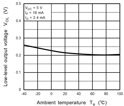
Fig. 13.2.10 V_{OL} - T_a
