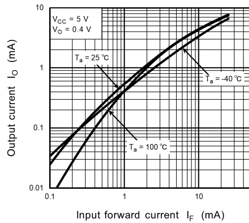
Fig. 13.2.4 I_O - I_F
