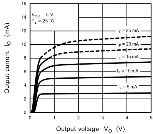
Fig. 13.2.8 I_O - V_O
