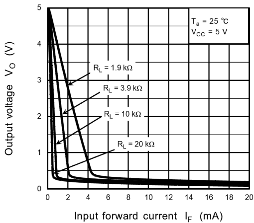
Fig. 13.2.9 V_O - I_F
