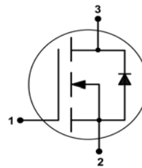
PG-SOT323
