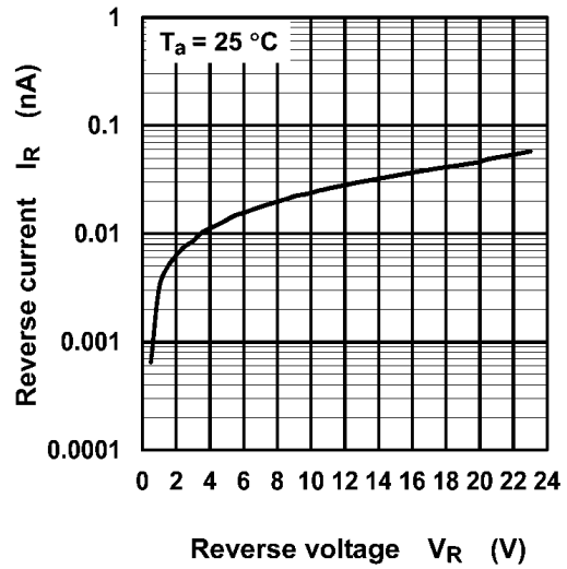
Fig. 8.2 I_R - V_R
