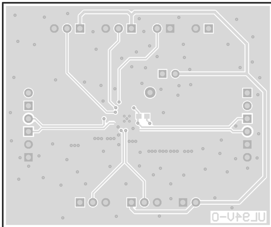
Figure 4-6. Bottom Layer
