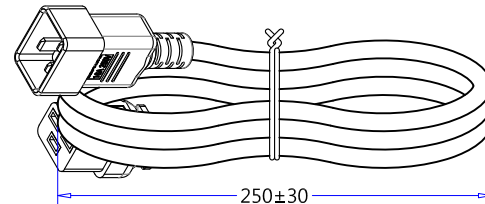
B-C3 扎線圖示 (Tied Loop Hank Detail)
