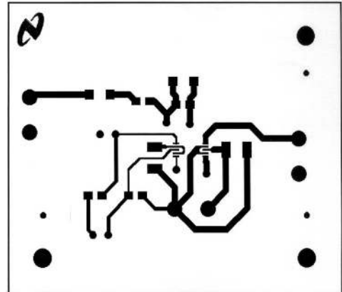
Top Layer
