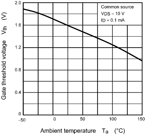
Fig. 7.7 V_{th} - T_a
