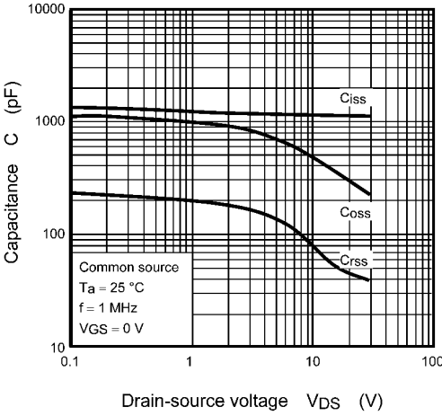
Fig. 7.9 C - V_{DS}
