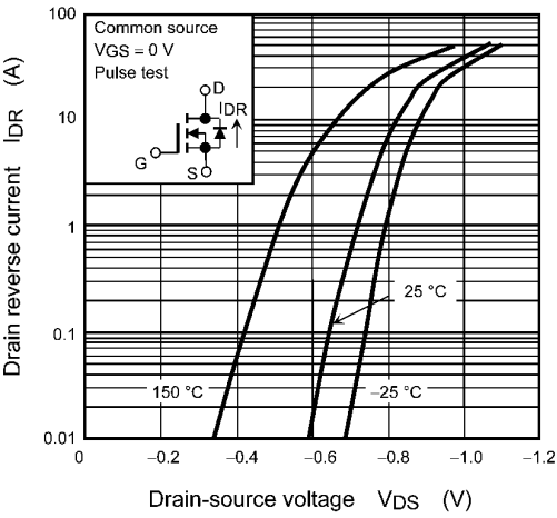
Fig. 7.8 I_{DR} - V_{DS}
