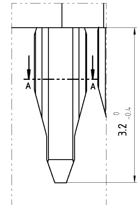
Einzelheit H (20:1) Detail H (20:1)
