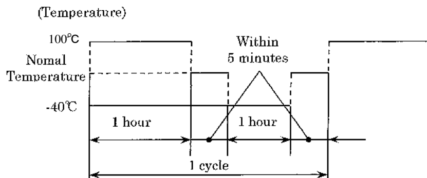
Fig. 10 Thermal shock
