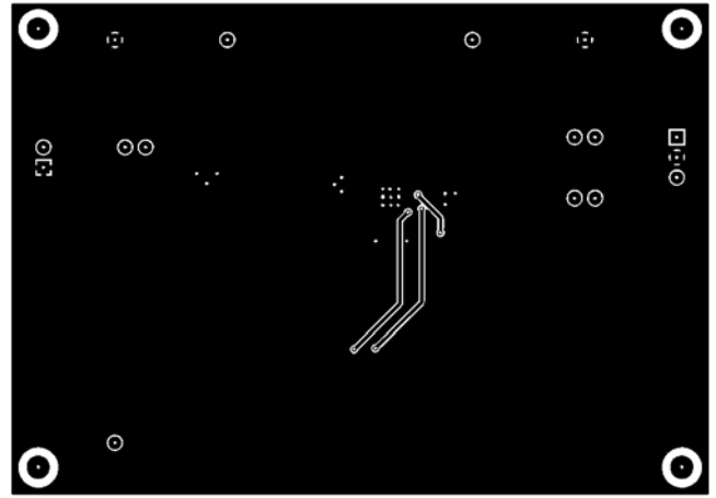
Bottom Layer
