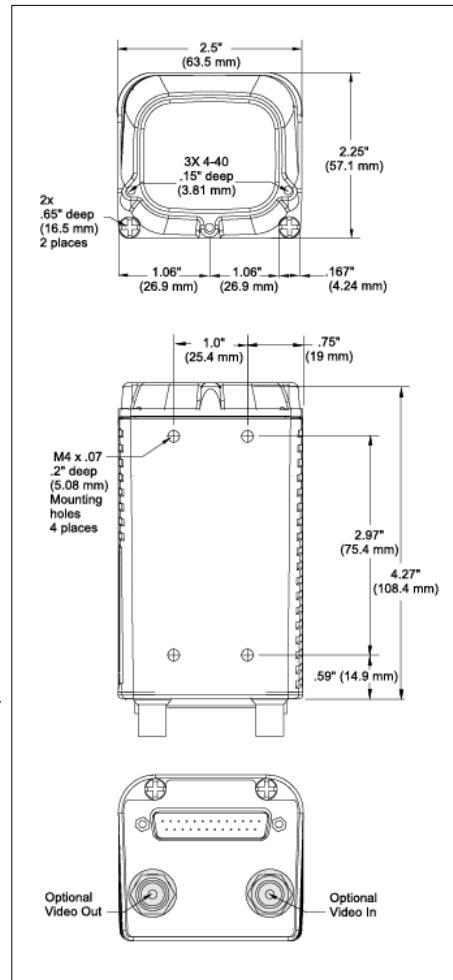
Quadrus EZ Reader Dimensions
