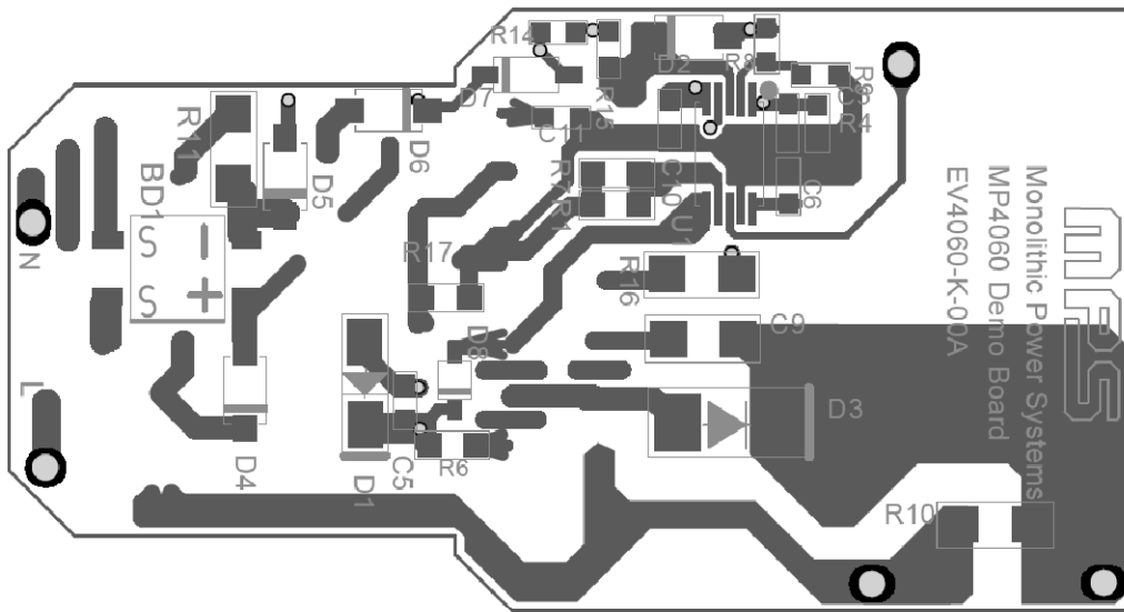
Figure 3—Bottom Layer
