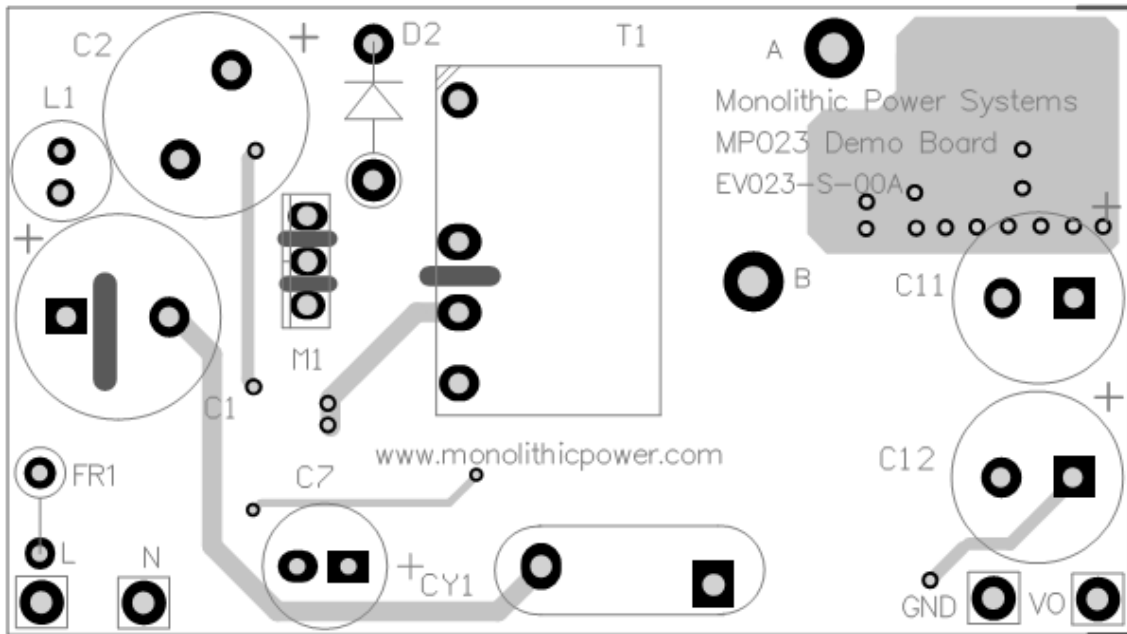
Figure 2—Top Layer
