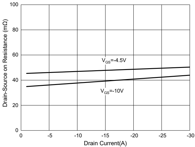
Fig. 10 - R_{DS(ON)} - I_D
