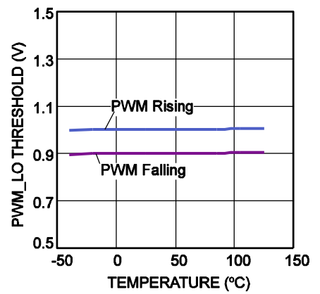
PWM Lo
