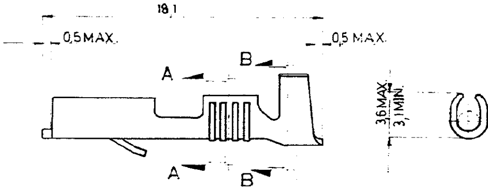
SECCION-A-A
