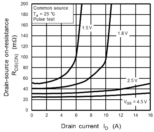
Fig. 7.1.4 R_{DS(ON)} - I_D
