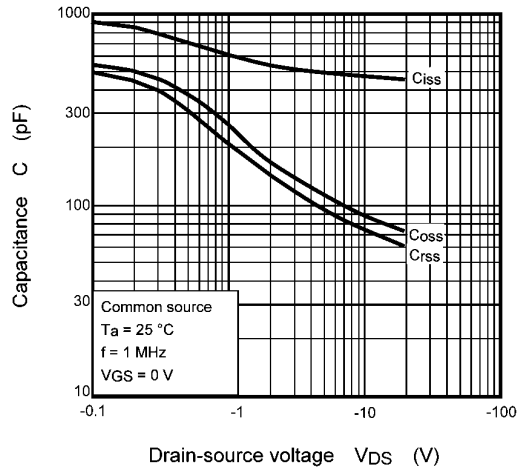
Fig. 7.2.10 C - V_{DS}
