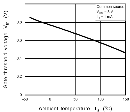
Fig. 7.1.6 V_{th} - T_a
