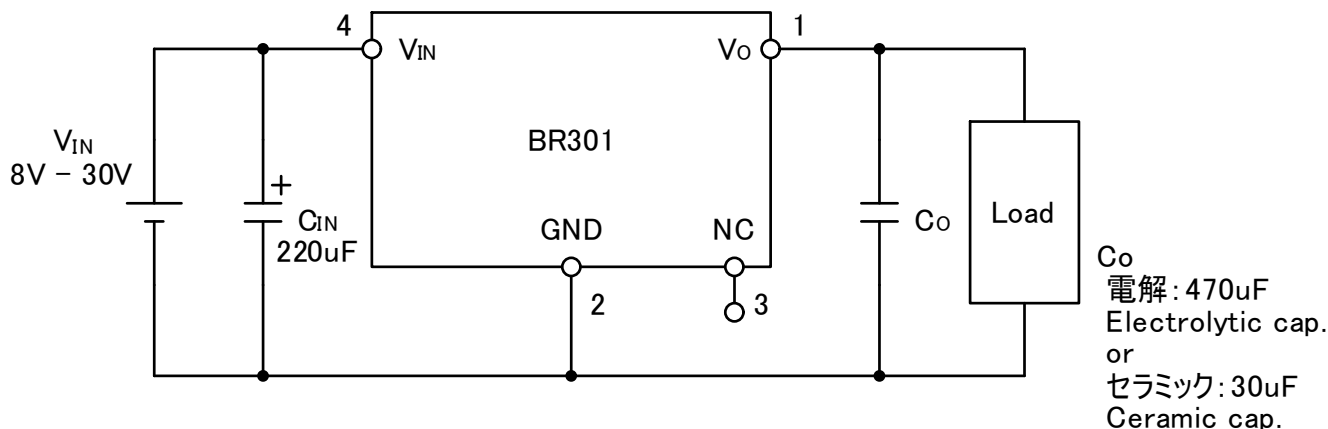
標準接続図
