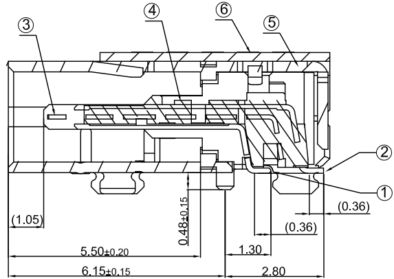
SECTION A-A(剖视图A-A) SCALE 2:1 (比例 2:1)
