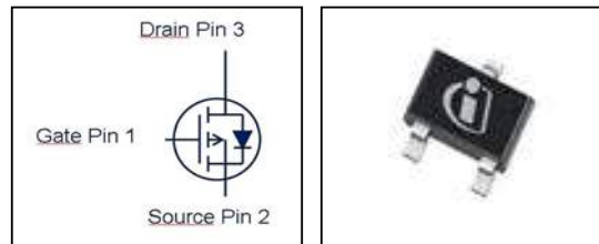
PG-SOT-323
