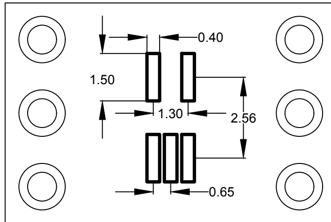
Back: SOT353
