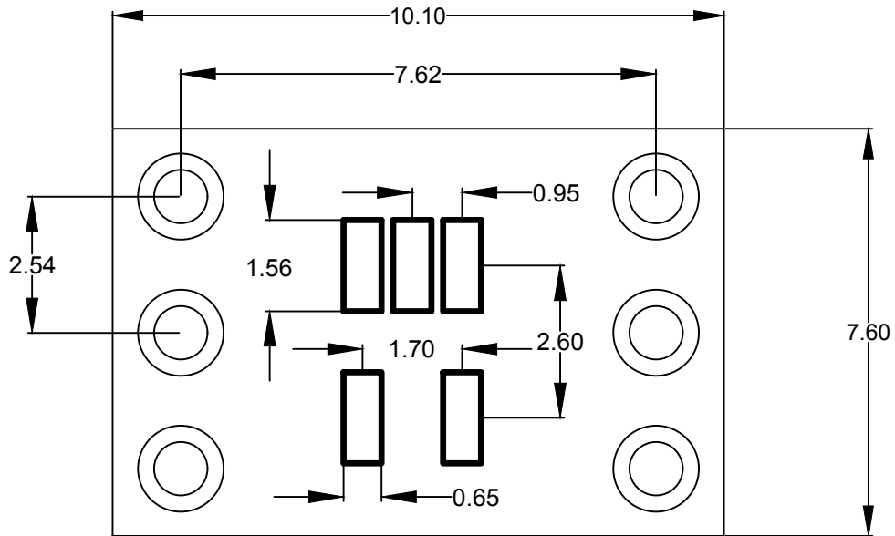
Front: SOT23-5
