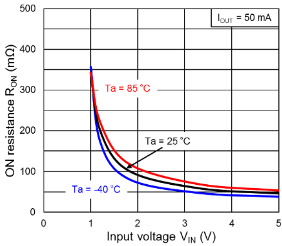
R_{ON} - V_{IN}
