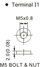
[M5 BOLT & NUT]
