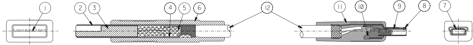
USB A
