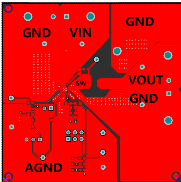
Figure 4-2. Top Layer
