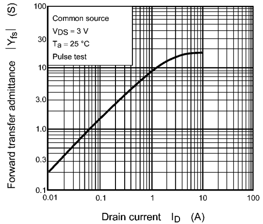
Fig. 8.8 |Y_{fs}| - I_D
