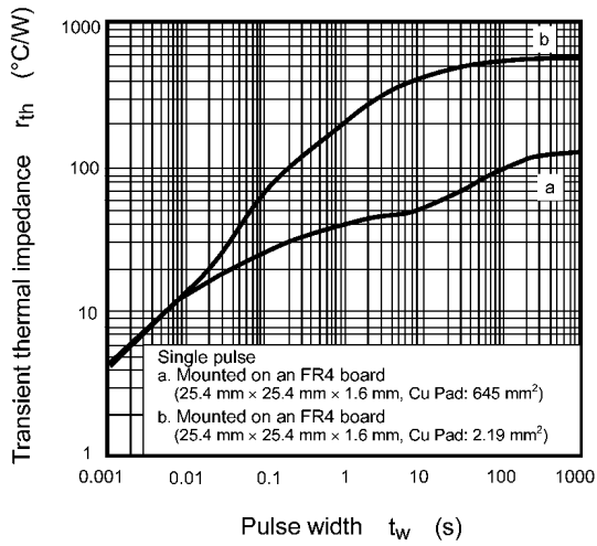
Fig. 8.13 r_{th} - t_w
