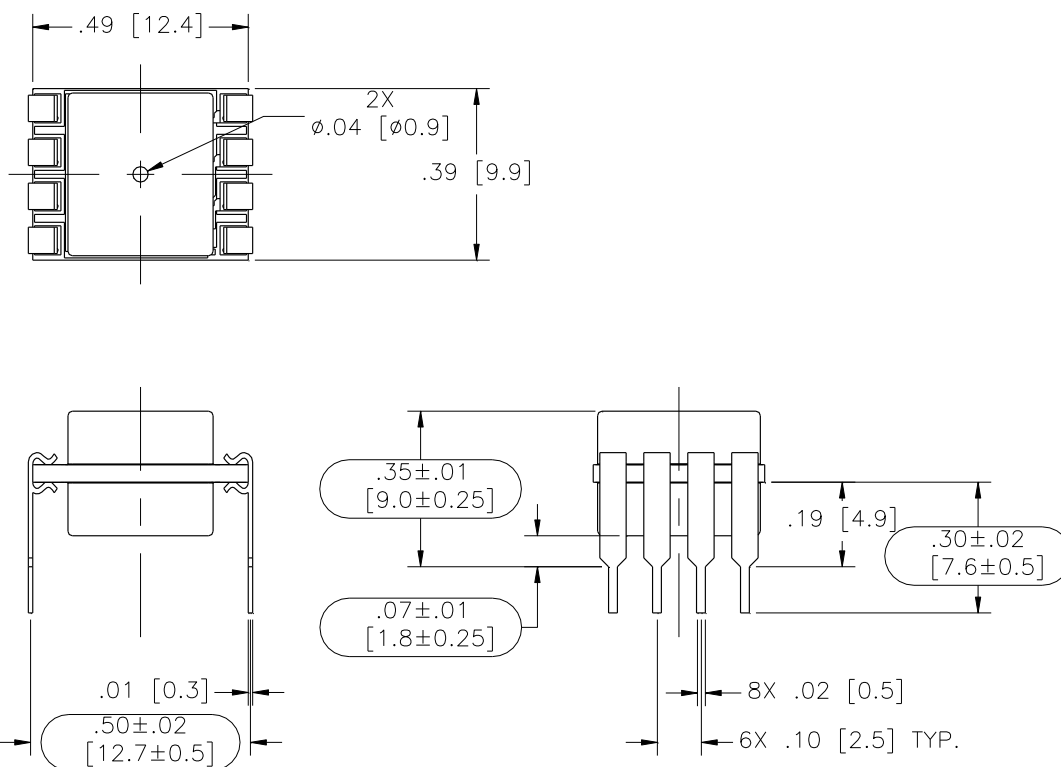
Model: MS4525-MMvoxxxP
