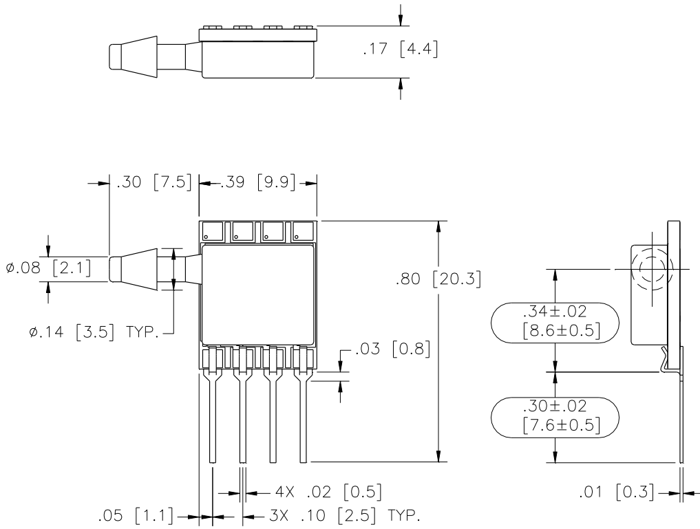
Model: MS4525-SSvoxxxxL
