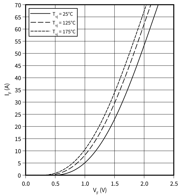
Durchlasskennlinie der (typisch), Diode, Brems-Chopper
