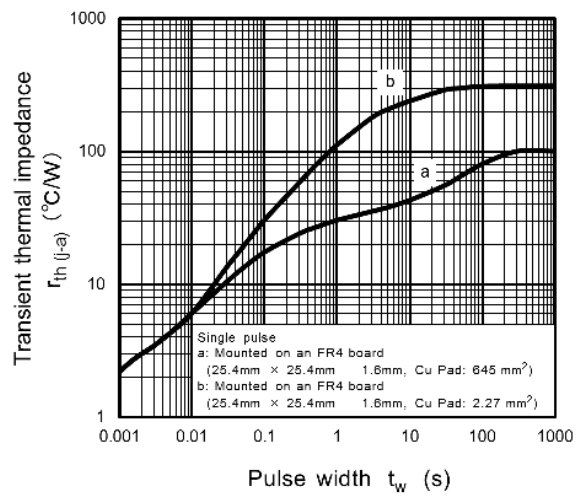
Fig. 8.6 r_{th} - t_w
