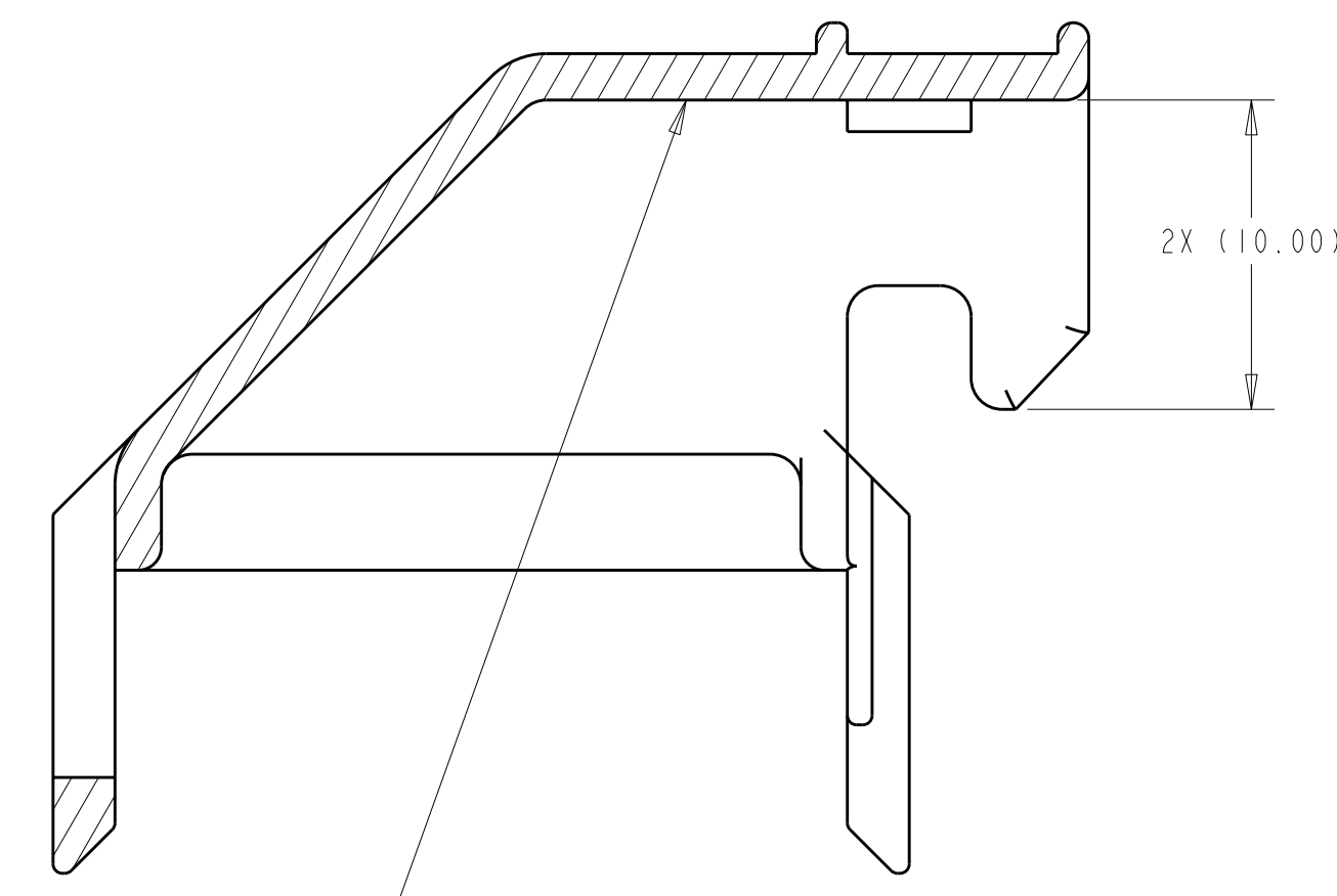
SECTION A-A
