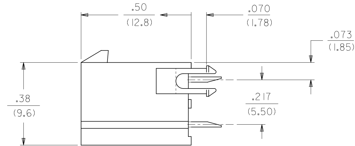
8 CKT SHOWN
