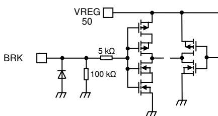
13) BRK pin
