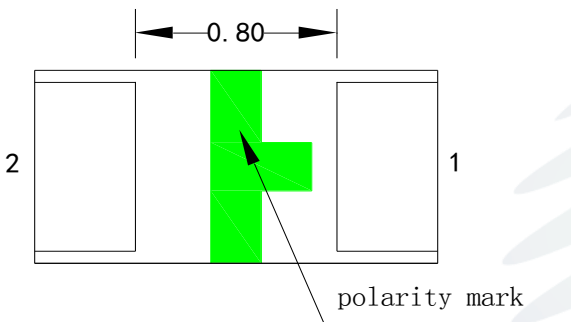
Fig.1-3 Bottom view 背面视图
