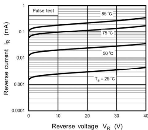
Fig. 9.2 I_R - V_R
