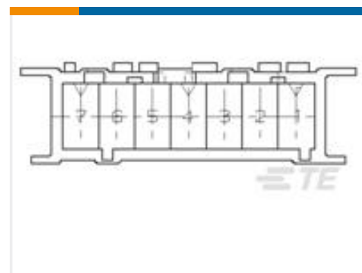
TE Part # 928309-7 7P FF FLACHST GEH
