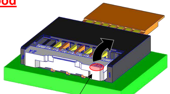
偏った部分での操作 Push up the one side of actuator
