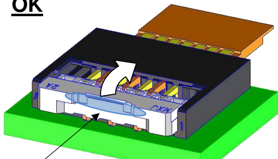
アクチュエータ下面中央部を操作 Push up the center bottom area of actuator
