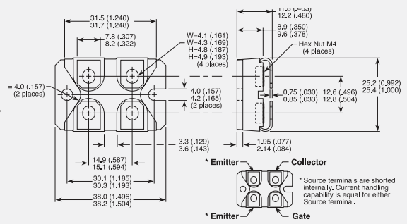
SOT-227
