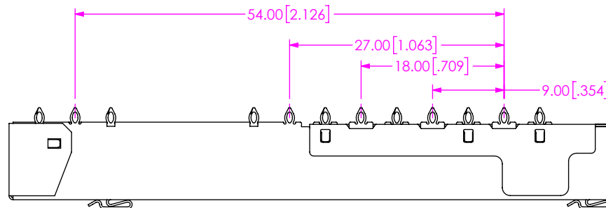
FIG 1 QSFP-DD-1-1-S-F SHOWN
